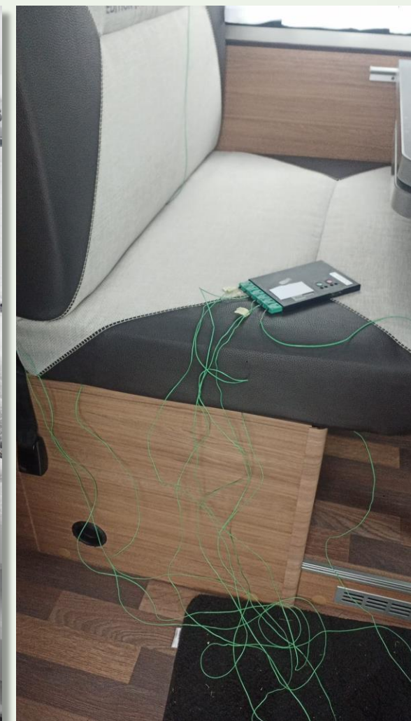
Datapaq zur Temperaturmessung
